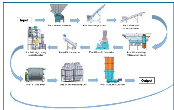
Fig. 4 : Flow-sheet pour une installation de lavage pour films agricoles
