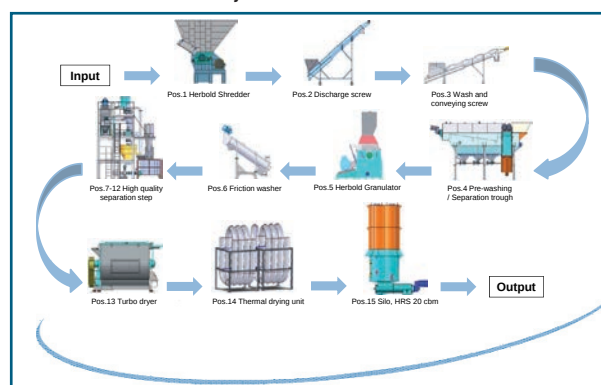
Foto/Fig.4: Esquema de flujo para una instalación de lavado para folio agrícola
