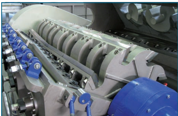
Foto/Fig. 1: Molino de corte SMS de la serie SB con alimentación forzada
