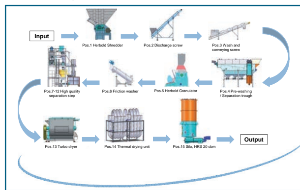
Abb. 4: Flow-Sheet für eine Waschanlage für Landwirtschaftsfolie
