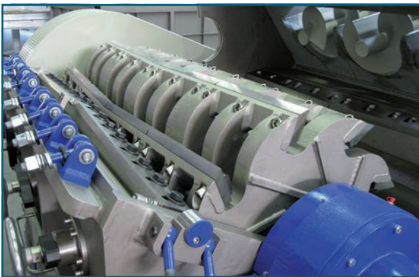
Abb. 1: Schneidmühle SMS Baureihe SB mit Zwangsbeschickung
