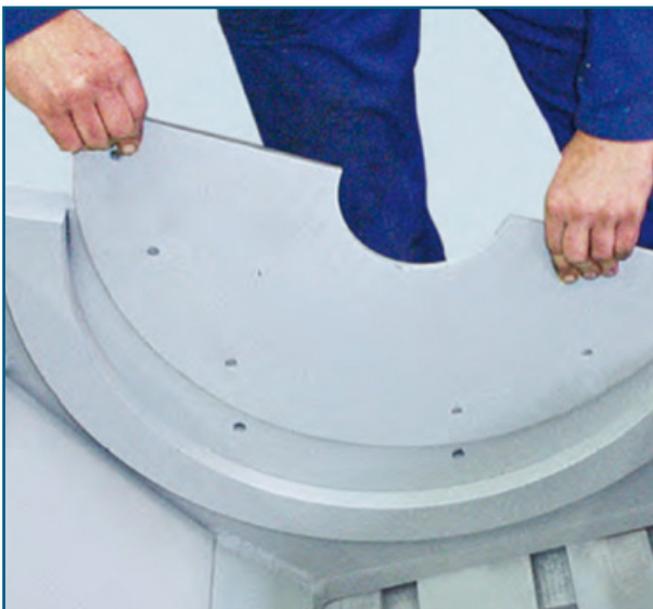
Рис. 1: Дробильная камера всех ножевых дробилок полностью защищена с помощью сменных износостойких пластин.
