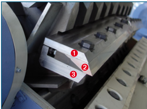
Рис. 3: ❶ прижимная планка ножа ❷ нож ротора ❸ сменная деталь, защищающая от износа
