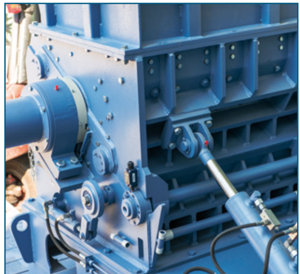
Рис. 2: Сменные износостойкие пластины прикручены снаружи.
