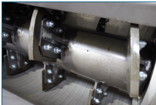
Рис. 8: Сменная лопасть, подверженная износу
