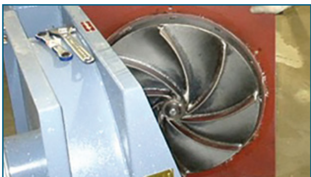
Рис. 7: Крыльчатка воздуховодки имеет изогнутые лопатки, которые уменьшают износ и предотвращают нежелательное доизмельчение материалов внутри воздуховодки. Может поставляться из высококачественной стали в качестве серии EHST.
