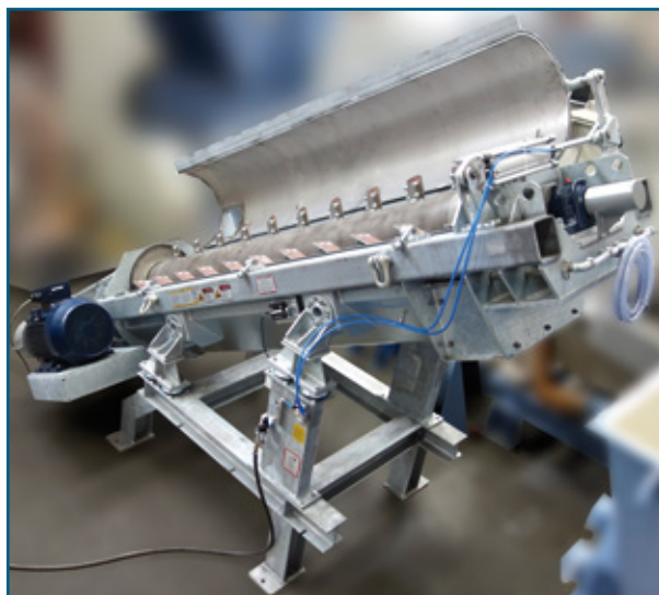
Рис. 9: Пневматическое открытие корпуса, обеспечивающее доступ для проведения технического обслуживания, сокращение времени простоев
