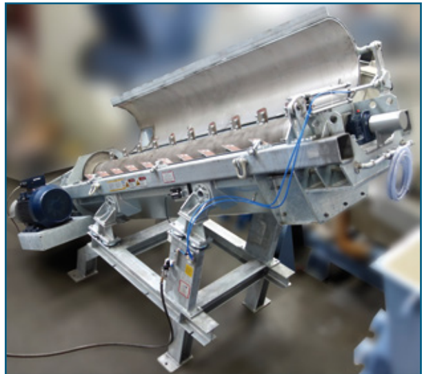
Fig. 9 : Ouverture pneumatique pour les travaux de maintenance, réduction des temps d'arrêt.
