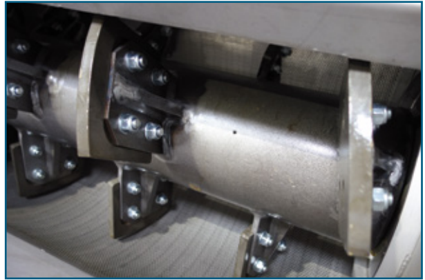
Fig. 8 : Pale d'usure échangeable
