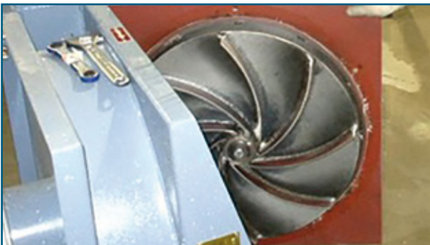
Foto/Fig.7: La rueda del soplador dispone de palas curvas que disminuyen el desgaste evitando además una trituración posterior del material dentro del soplador. También puede suministrarse de la serie EHST de acero para altos rendimientos.
