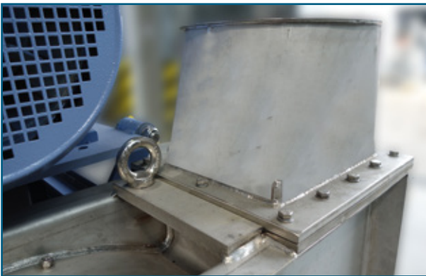
Foto/Fig.6: ... así como de manguitos de aspiración y presión también recambiables.
