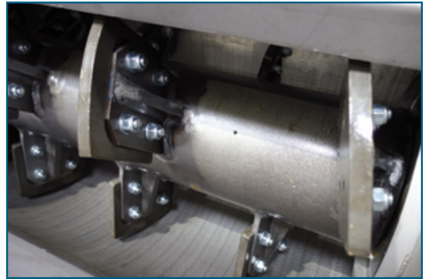
Foto/Fig.8 : Paletas antidesgaste recambiables
