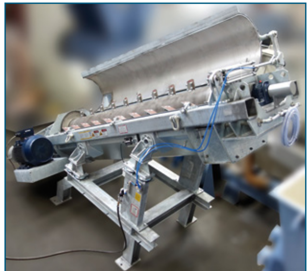
Foto/Fig.9: Apertura neumática para mantenimiento, reducción de tiempos de paro.
