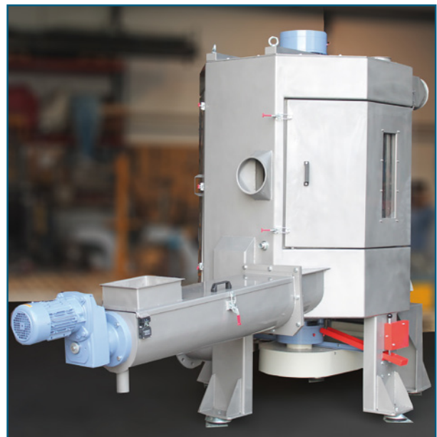
Рис.1: Гербольд Сушилка HVT 90-150
