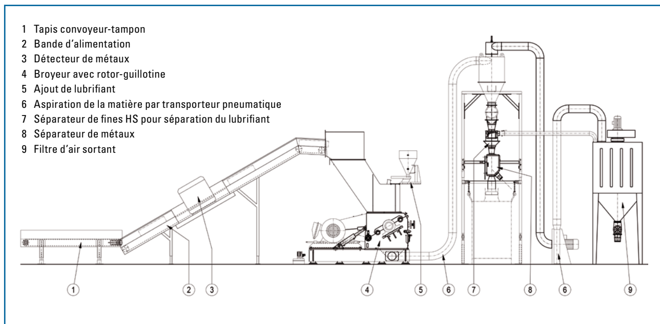
Broyage simple avec entrée et récupération de talc
