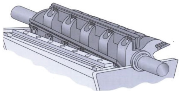
Fig. 2: Corte doble inclinado
