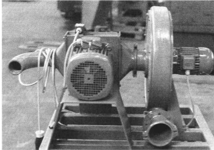
Modèle spécial SML 20/10 AD pour le recyclage de lisières de feuille
