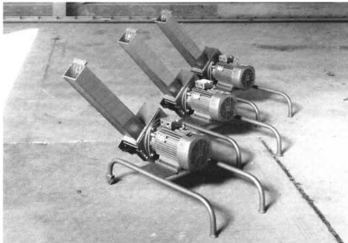
Modèle spécial SML 20/10 pour le broyage de tuyaux et profilés
