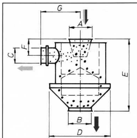
séparateur de fines HS
