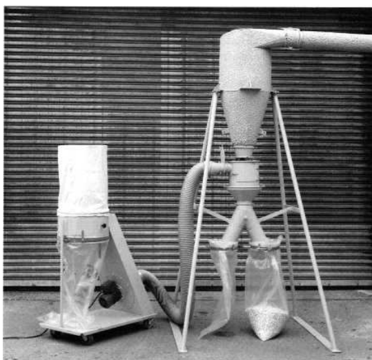
cyclone séparateur avec séparateur de fines HS 300 (récupération en sacs)
