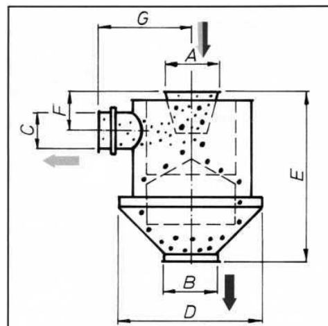
Prinzipzeichnung Feingutabscheider HS
