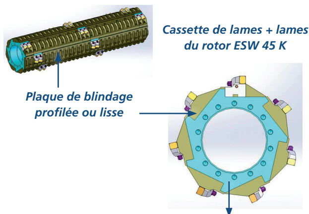
Illustration du rotor
