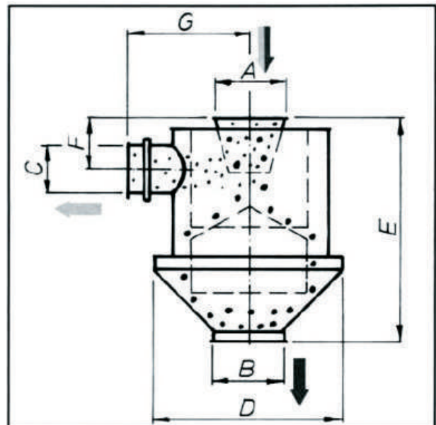
Prinzipzeichnung Feingutscheider HS
