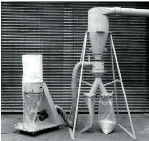
Zyklonabscheider mit Feingutscheider HS 300 (Absackausführung)
