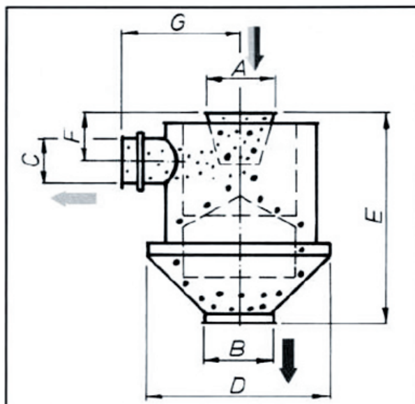
Принципиальный чертеж сепаратор мелких фракций HS
