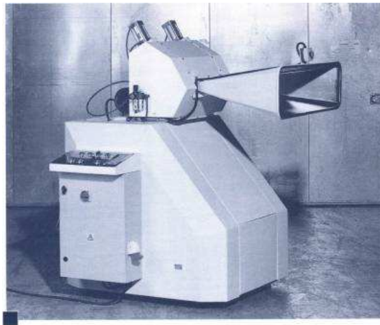
SML 35/42 с интегрированной звуковой изоляцией, питающим валком и бункером сбора
