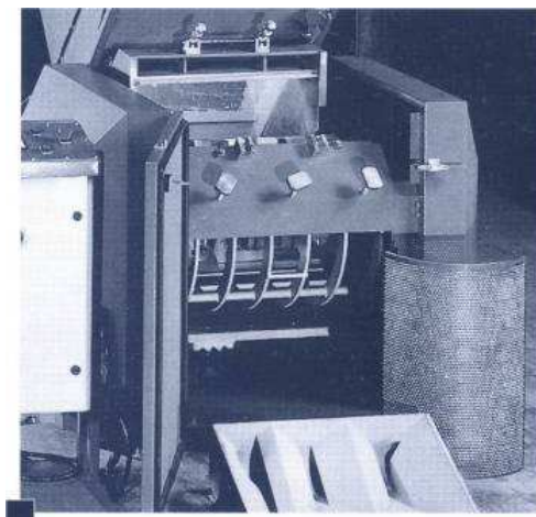
Легкий доступ в камеру дробления
