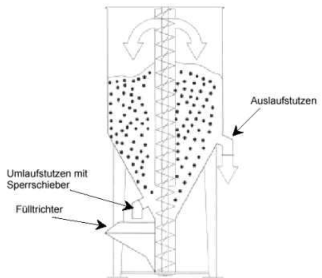
Funktionsschema
