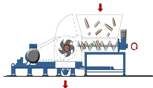
Prinzipskizze: Herbold Schneidmühlen Baureihe SB
